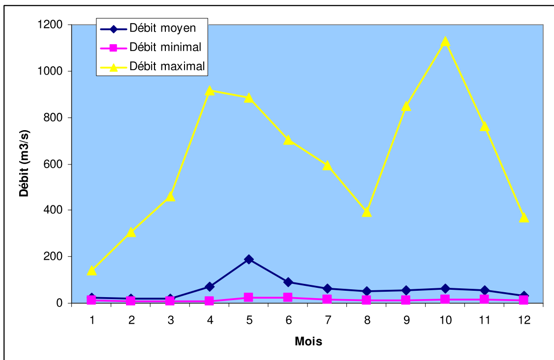
Figure 55. Débits moyens mensuels de la rivière Jacques-Cartier entre 1924 et 2008
